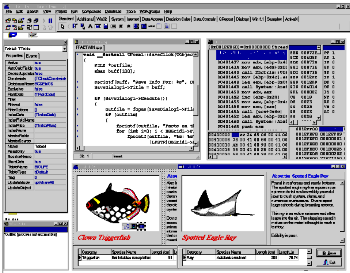
Den avancerade utvecklingsmiljön i C++ Builder 3 under debugging av ett databasprojekt
